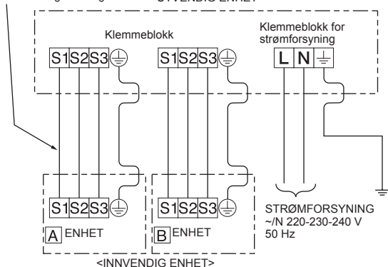
Koblingsledning mellom innvendig/utvendig enhet <UTVENDIG ENHET>
